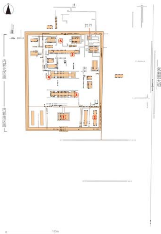
第4図 飛鳥宮遺跡第Ⅲ—A期遺構配置図
